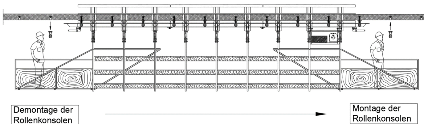
Brücken-Längsansicht
