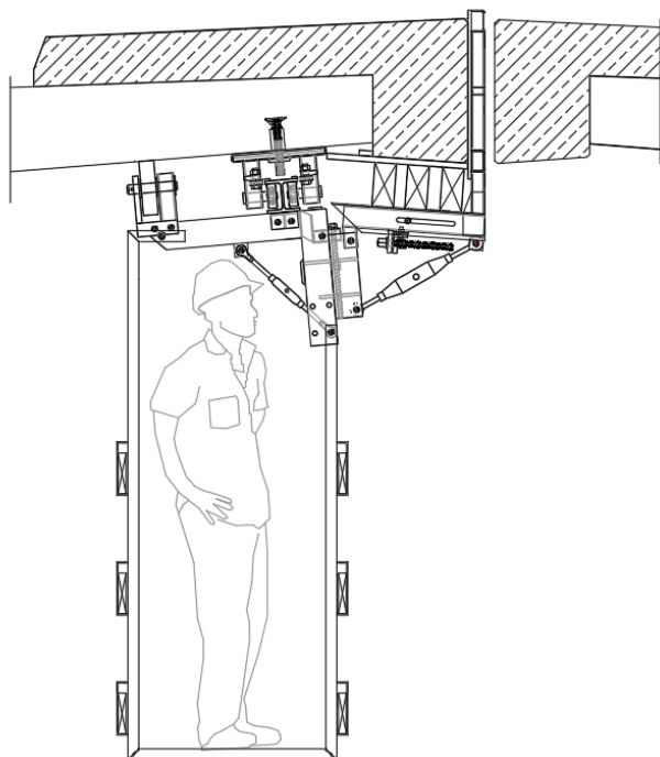
Brücken-Querschnitt
